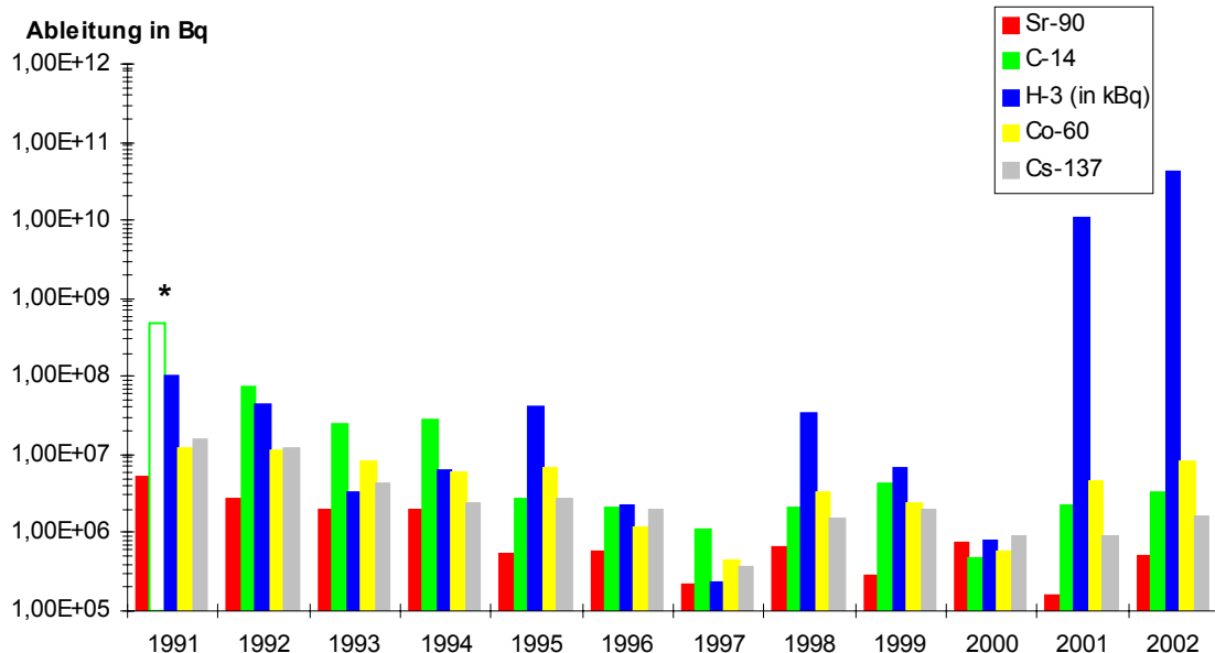
Abbildung 10: Ableitung expositionsrelevanter Radionuklide mit Wasser aus Rückhalteeinrichtungen des Forschungsstandortes Rossendorf 1991 bis 2002 /15/
