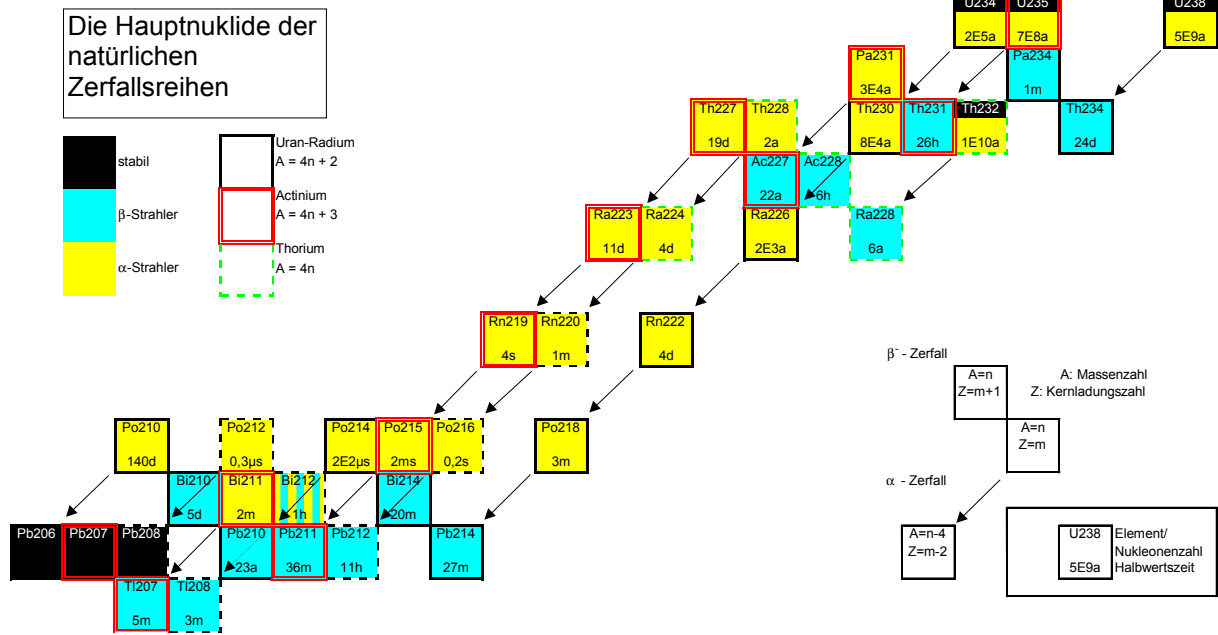
Abbildung 2: Schematischer Ausschnitt aus der Nuklidkarte mit den Hauptnukliden der natürlichen Zerfallsreihe
