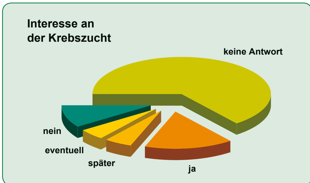
Abb. 69: Ergebnis der Umfrage unter 62 sächsischen Haupteinwerbungs-Fischereiunternehmen zu ihrem Interesse an der Haltung von Flusskrebsen in der Aquakultur: Von den 22 zurückgesandten Fragebögen bekundeten 16 Unternehmen ein mehr oder weniger großes Interesse. Lediglich sechs Unternehmen waren überhaupt nicht interessiert.
