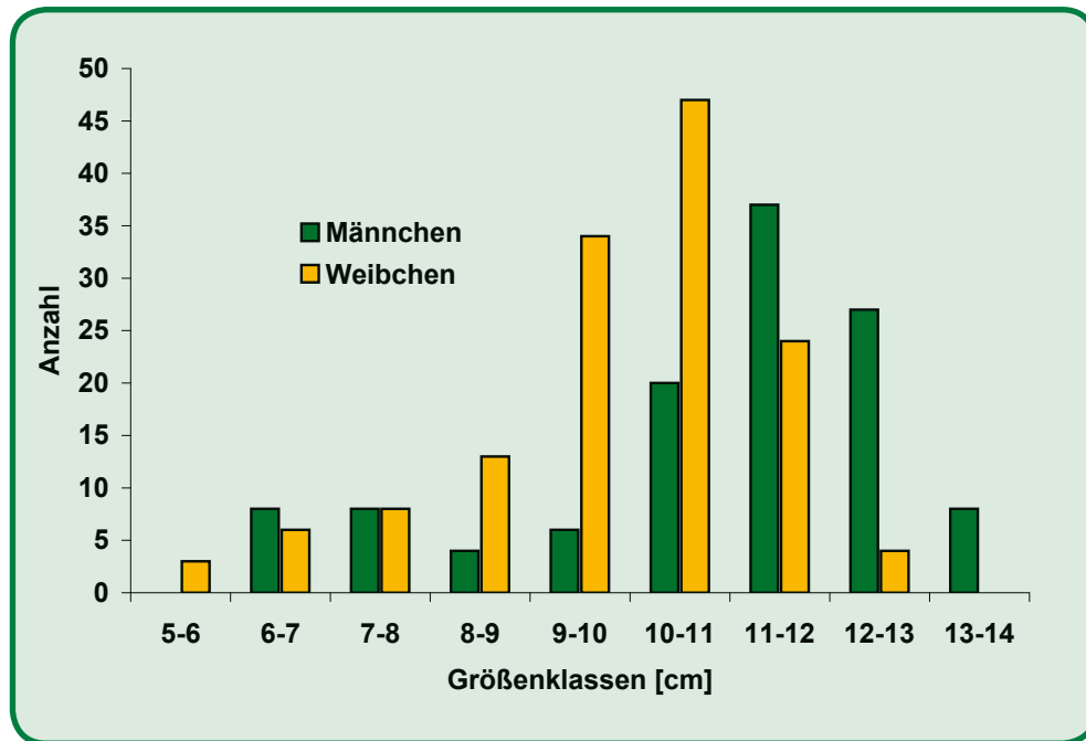
Abb. 62: Größenverteilung einer Edelkrebpopulation am Beispiel eines Teiches bei Chemnitz. Der Probenumfang betrug 118 Männchen und 139 Weibchen.
