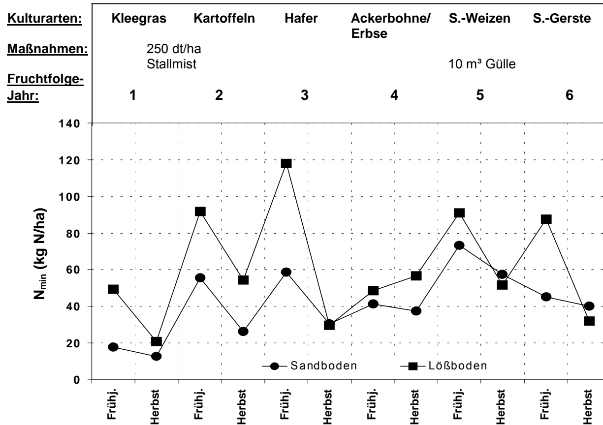
Abbildung 3: Verlauf der N_{\min} -Werte (kg N/ha, 0 – 90 cm Bodentiefe) in 6-feldrigen Fruchtfolgen mit Klee-gras sowie Körnerleguminosen (Ackerbohne auf Lößboden; Erbse auf Sandboden; ökologische Exaktversuche, Sachsen)
