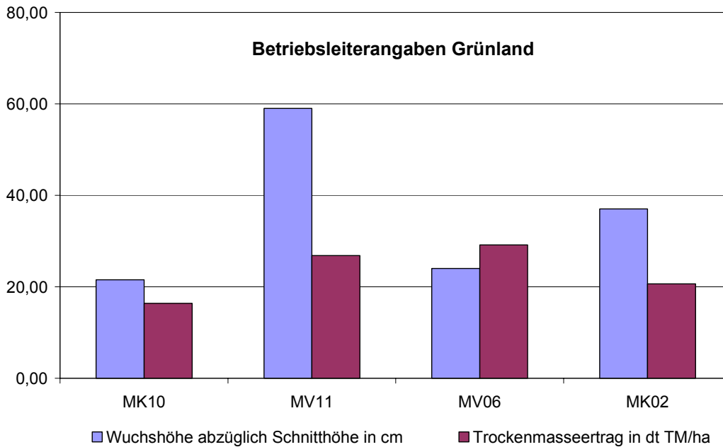
Abbildung 5: Abweichungen der Kennzahlen „Wuchshöhe abzüglich Schnitthöhe“ und „Gemessene TM-Erträge“ der Betriebsleiterangaben - Grünland, 1. Schnitt
