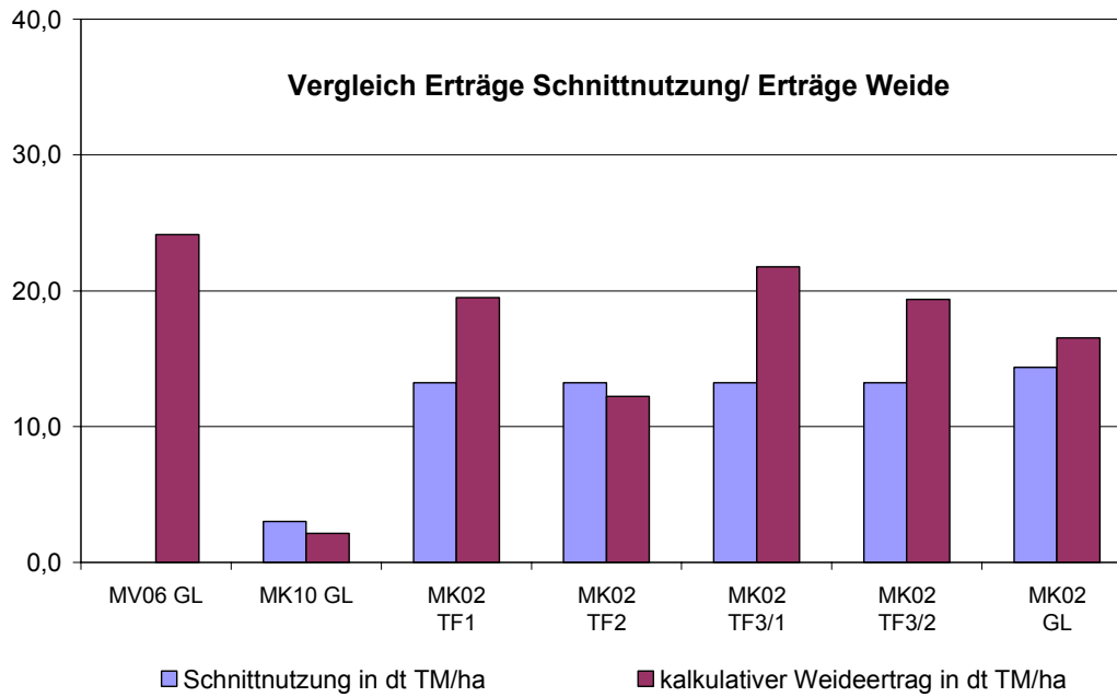
Abbildung 11: Vergleich der Erträge der Schnittnutzungen und der kalkulativen Weideerträge, 2. Schnitt/Nutzung
