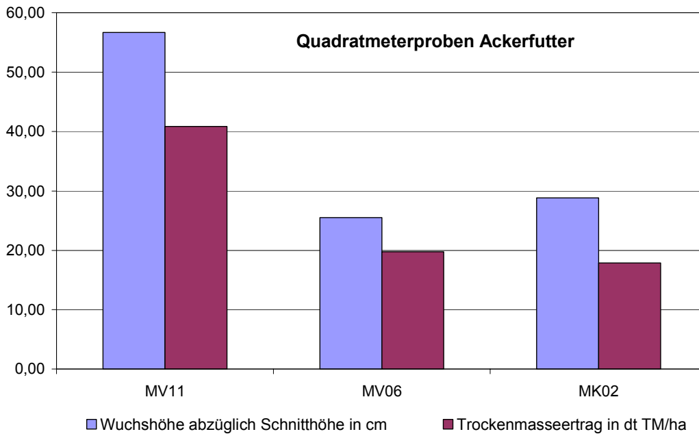
Abbildung 7: Abweichungen der Kennzahlen „Wuchshöhe abzüglich Schnitthöhe“ und „Gemessene TM-Erträge“ der m 2 -Proben – Ackerfutter, 2. Schnitt
