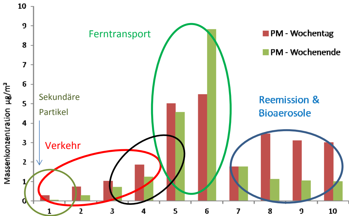
Abbildung 50: Partikelmasse für Wochenende und Wochentag und Zuordnung der Hauptquellen zu den Größenfraktionen des 10-stufigen Impaktors für je 2 Tagesmessungen in LEI im Herbst 2010
