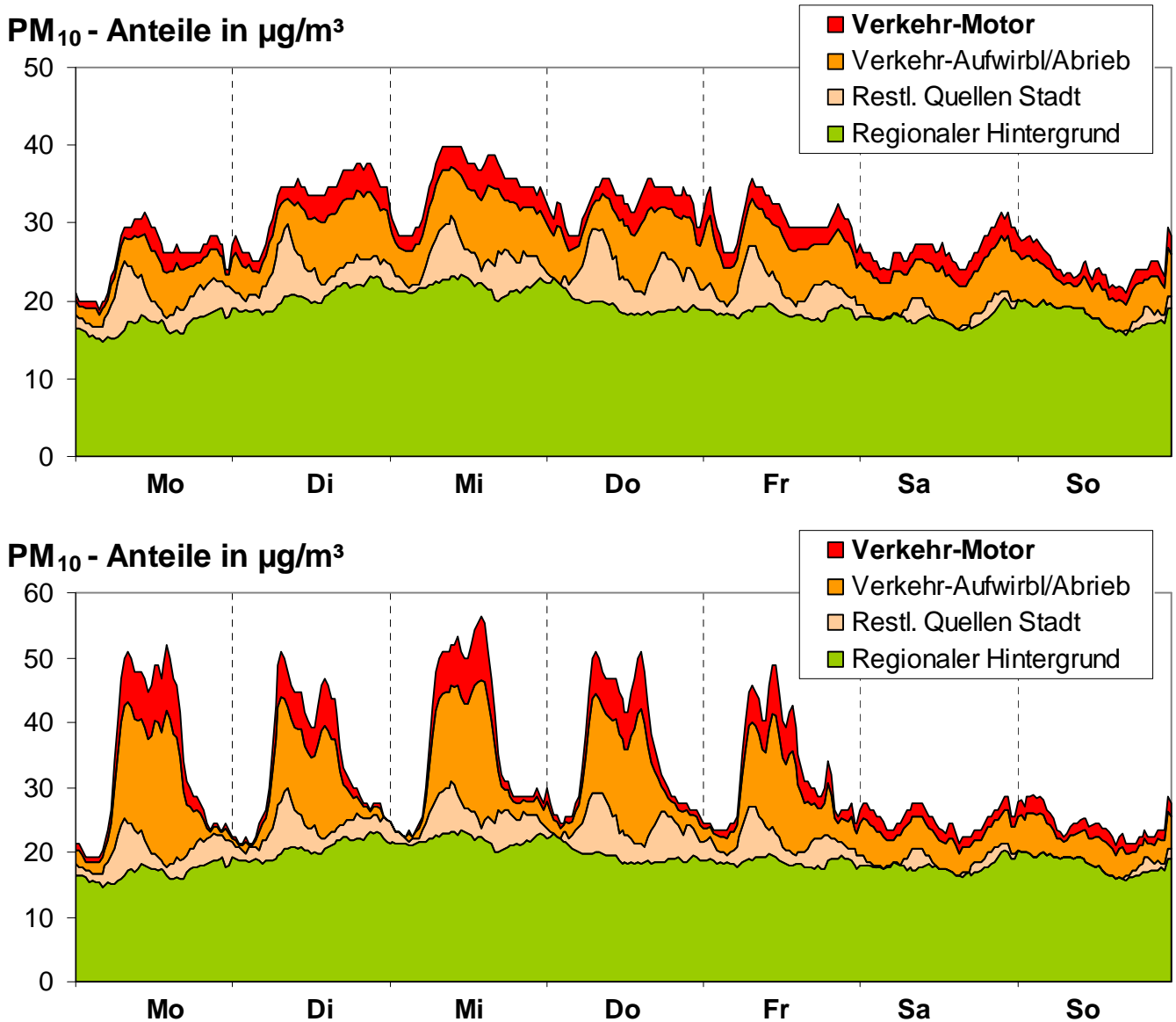
Abbildung 40: Mittlerer Wochengang für PM 10 im Jahr 2010 mit Verursacheranteilen an den verkehrsnahen Messstellen DDN (oben) und LMI (unten)
