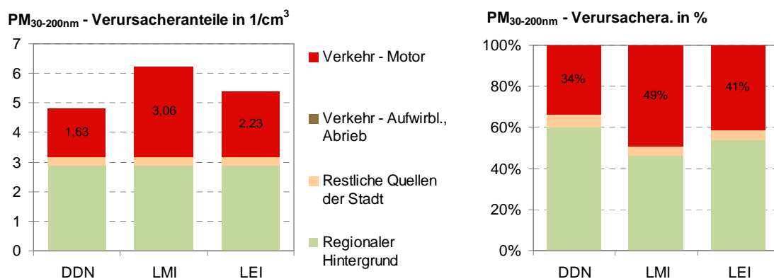
Abbildung 21: Anteile der Hauptverursacher für die aus der Partikelanzahl berechnete Partikelmasse PM 30-200 nm im Jahr 2010
