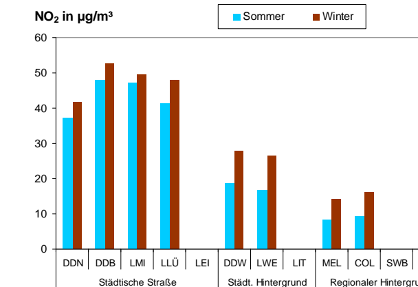
Abbildung 43: Vergleich der Mittelwerte für Sommer und Winter 2010 (oben Kfz-Zahlen, darunter Schadstoffe PM 10 , PM 2.5 Ruß EC , Ruß BC und unten PN 30-200nm bzw. NO 2 )
