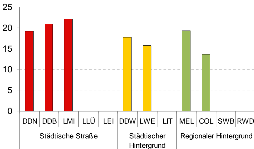
Abbildung 8: PM_{2.5} -Jahresmittelwerte 2010
