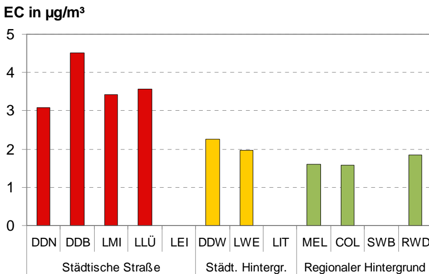
Abbildung 9: Orientierende Ruß EC -Jahresmittelwerte im PM 10 2010
