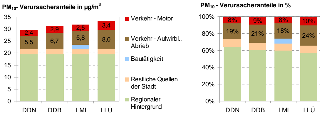
Abbildung 16: Anteile der Hauptverursacher für PM 10 im Jahr 2010 an den verkehrsnahen Messorten
