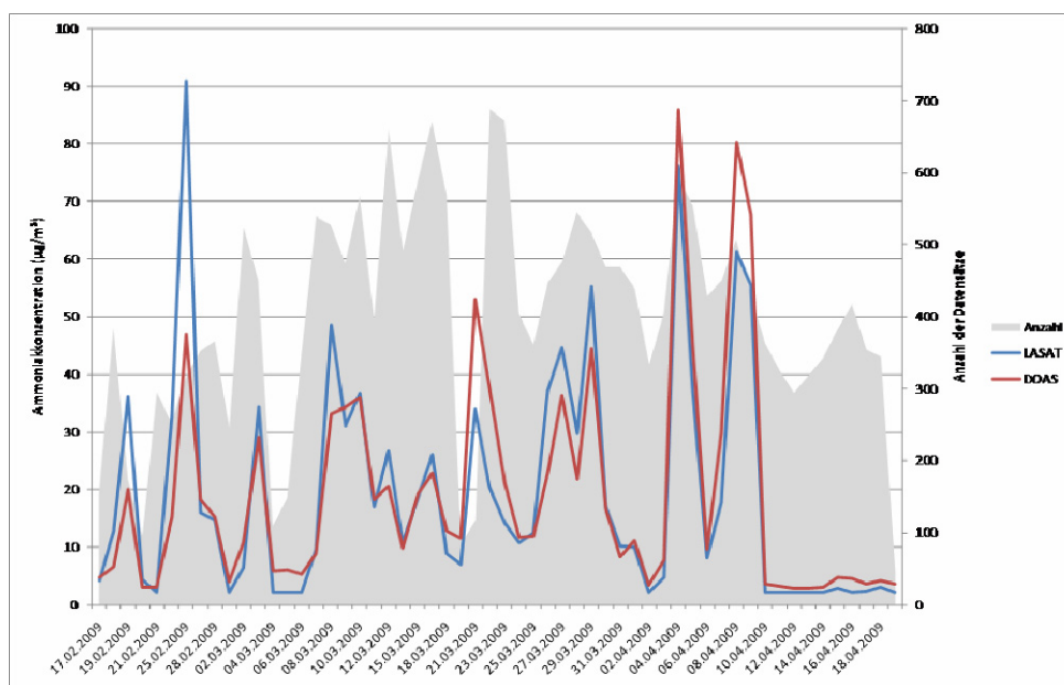
Abbildung 57: Betrieb 2 – Gegenüberstellung von LASAT-Immissionskenngrößen und DOAS-Messwerten für Episode 26 bei minutengenauer Herangehensweise
