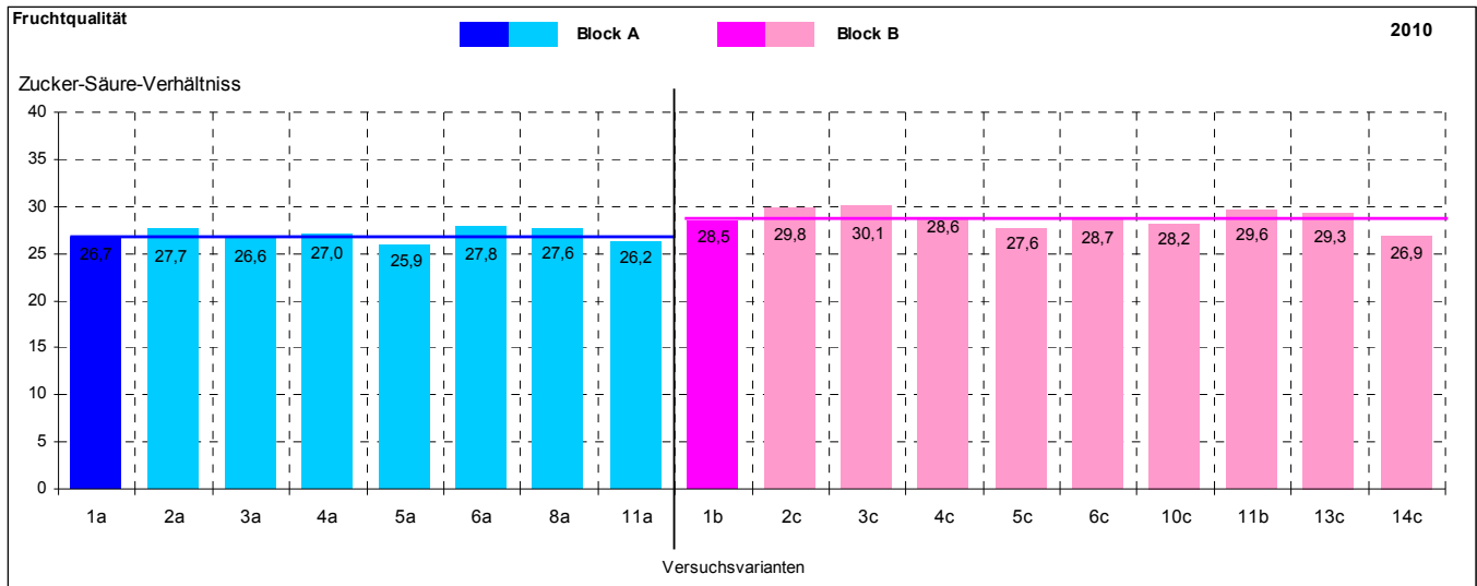
Abbildung 10: Berechnetes Zucker-Säure-Verhältnis, 2010
