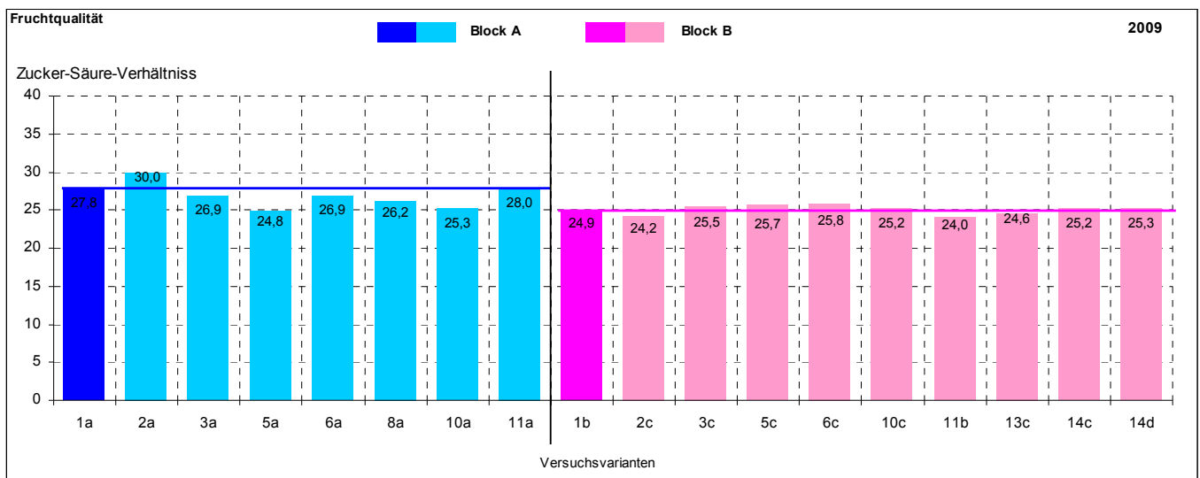
Abbildung 8: Berechnetes Zucker-Säure-Verhältnis, 2009
