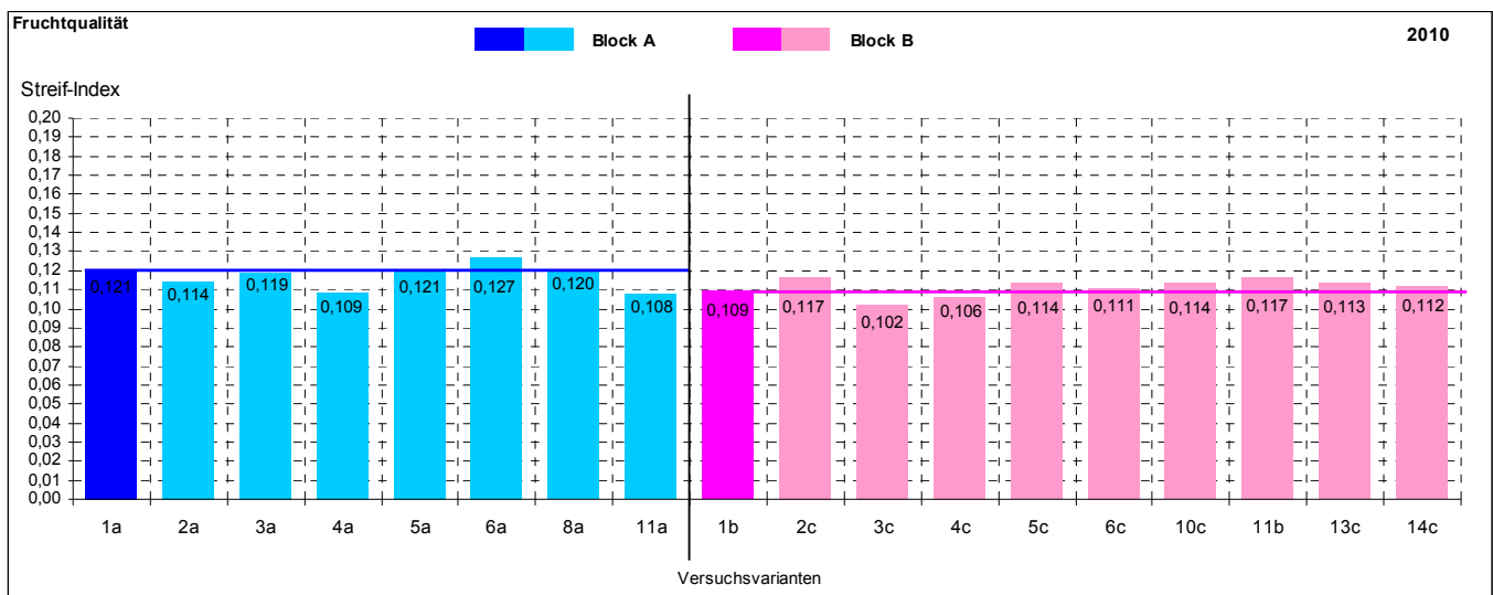
Abbildung 11: Berechneter Streifindex, 2010
