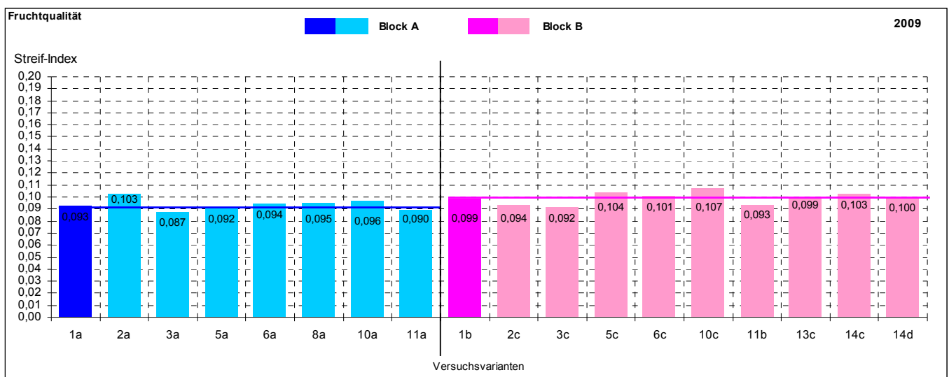
Abbildung 9: Berechneter Streifindex, 2009
