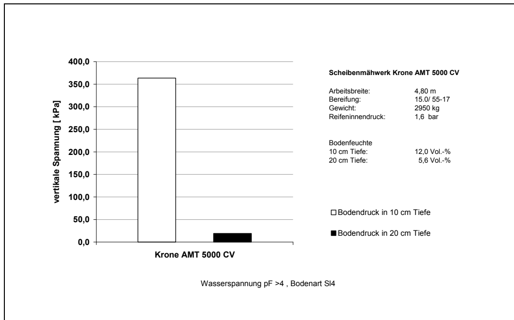
Abbildung 6: Vertikale Bodenspannungen (am 22.05.07) auf einer Grünlandfläche des LVG Köllitsch beim Mähen unter den Tragrädern des Mähwerkes in 10 cm und 20 cm Tiefe; detaillierte Angaben zu den Maschinen s. Anhang Tab. 21
