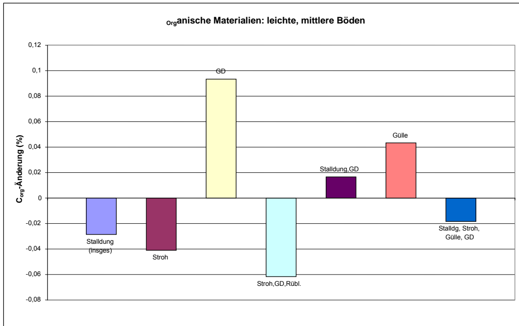
Abbildung 12: Abweichungen der C org -Gehalte am Versuchsende für das CCB-Verfahren von den im Feld gemessenen Gehalten für die Faktoren Stallung, Stroh, Gründüngung, Gülle und Mischvarianten
