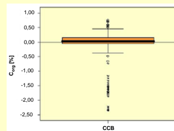
Abb.2: Median und Streubreite in den berechneten C_{org} -gehalten [%] des CCB-Verfahrens unter Einbeziehung aller praxisrelevanten Versuchsvarianten im Vergleich zu den jeweiligen Felddaten am Versuchsbeginn (= 0,0 %)
