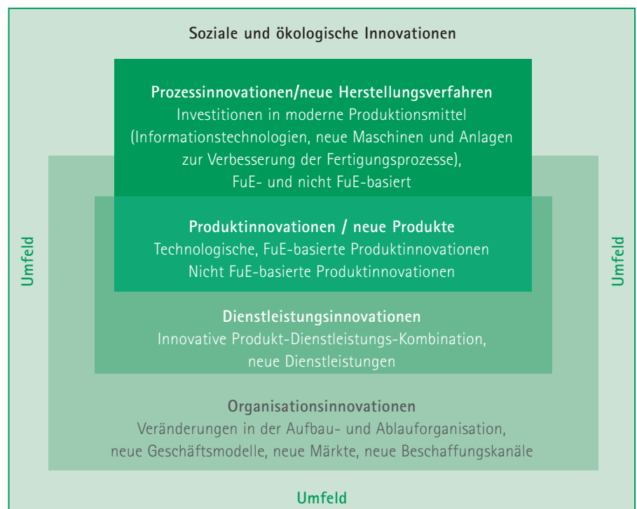
Abb. 3: Holistisches Innovationskonzept
