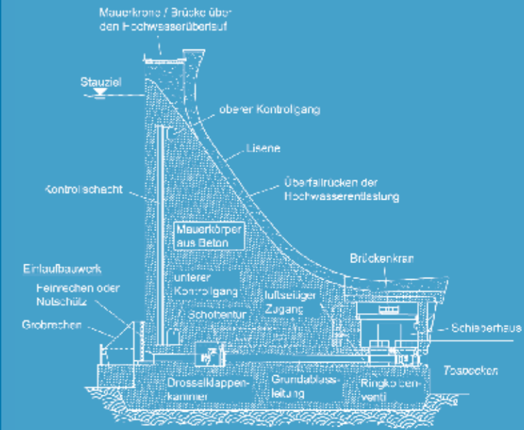
Querschnitt der Staumauer bei Grundablass und Hochwasserentlastung
