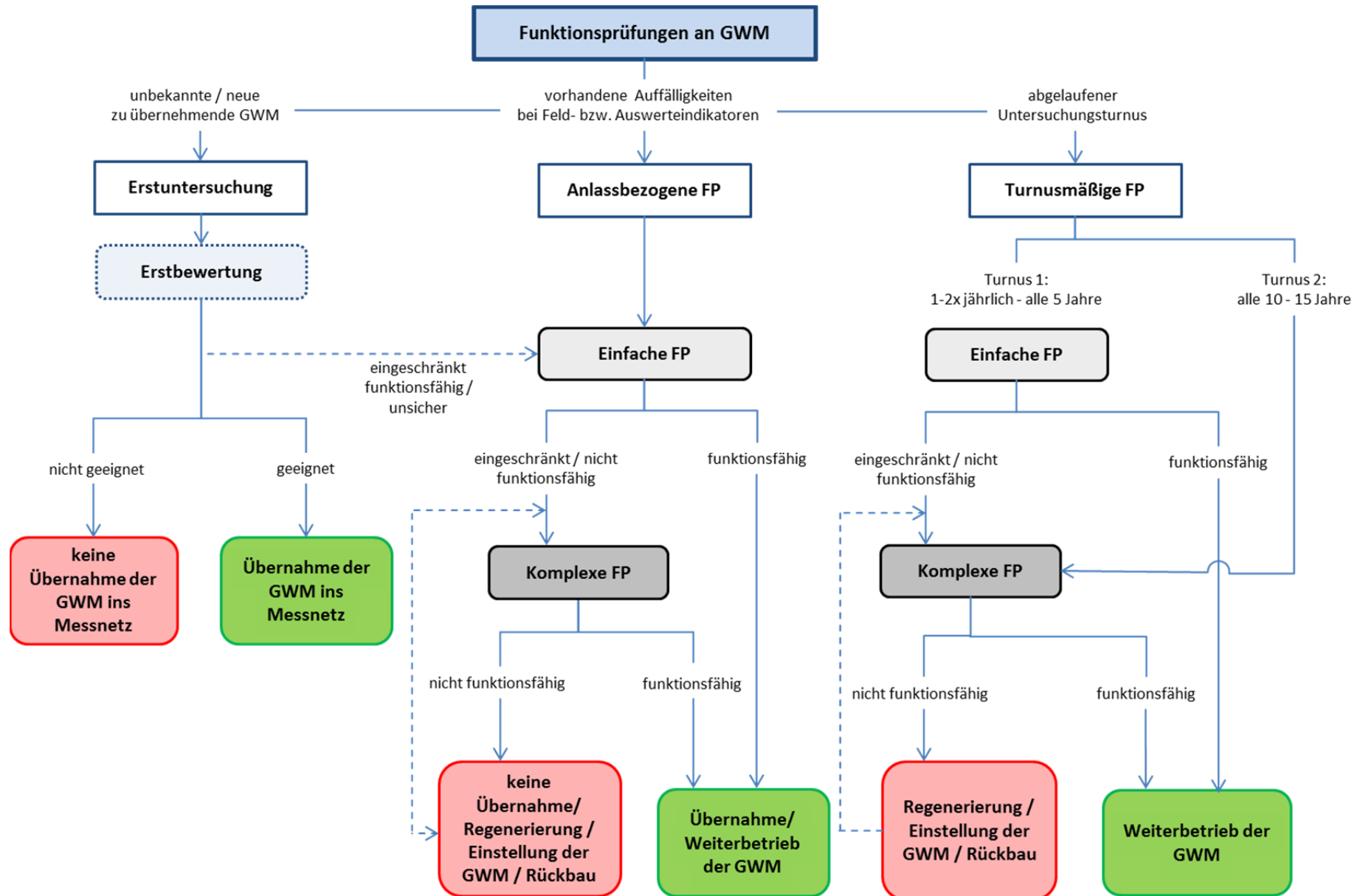
Abbildung 1-1: Entscheidungsablauf von Funktionsprüfungen an Grundwassermessstellen
