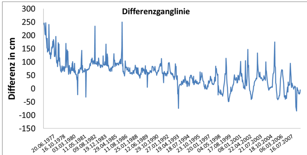
Abbildung 3-2: Differenzganglinie zweier Grundwassermessstellen
