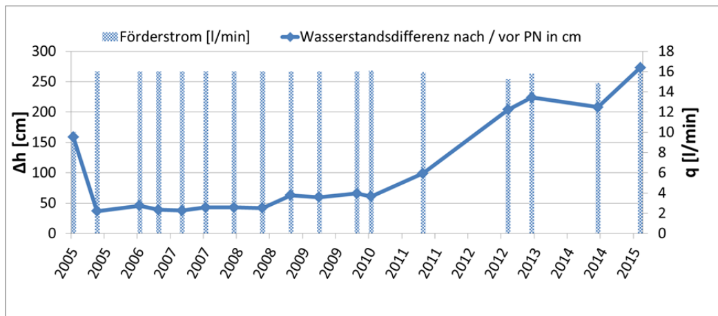
Abbildung 3-1: Entwicklung der Wasserstandsdifferenz \Delta h und des Förderstroms q bei einer Grundwasserprobennahme
