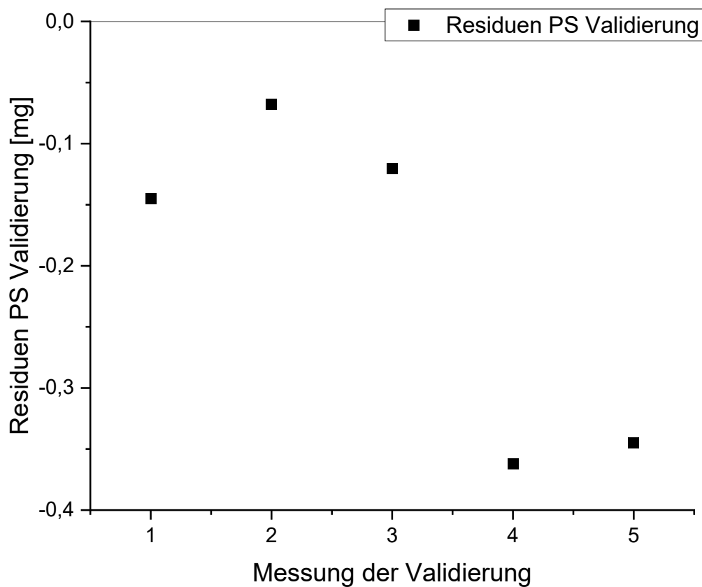
Abbildung 39: Residuen aus der Validierung der PS Kalibrierung
