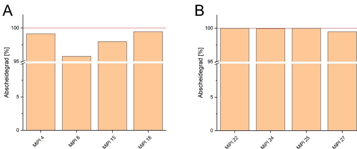
Abbildung 34: Abscheidegrade nach Dichteseparation von 2020 (A) und 2021 (B) elektroseparierten polymerreichen Fraktionen
