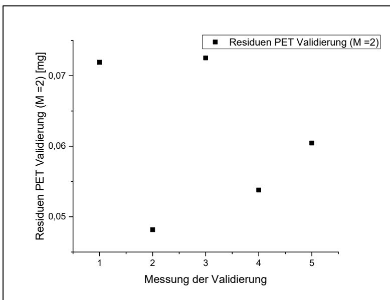
Abbildung 41: Residuen aus der Validierung der PET Kalibrierung
