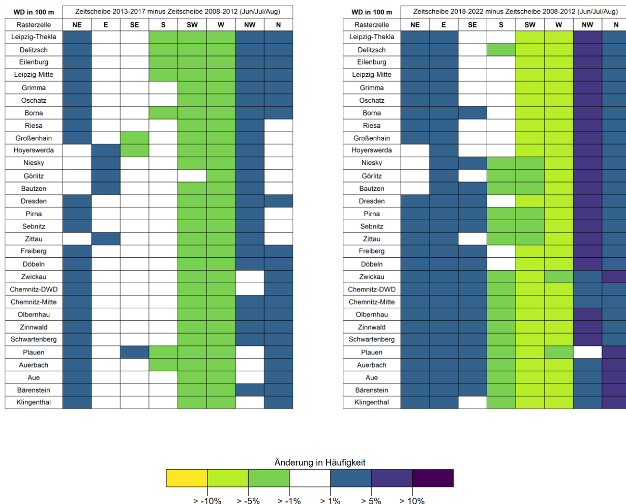
Abbildung 8: Unterschiede in der Windrichtungsverteilung für die Zeitscheibe 2013–2017 (links) sowie 2018–2022 (rechts) in Bezug auf die Zeitscheibe 2008–2012, jeweils für die Juni, Juli, August.
