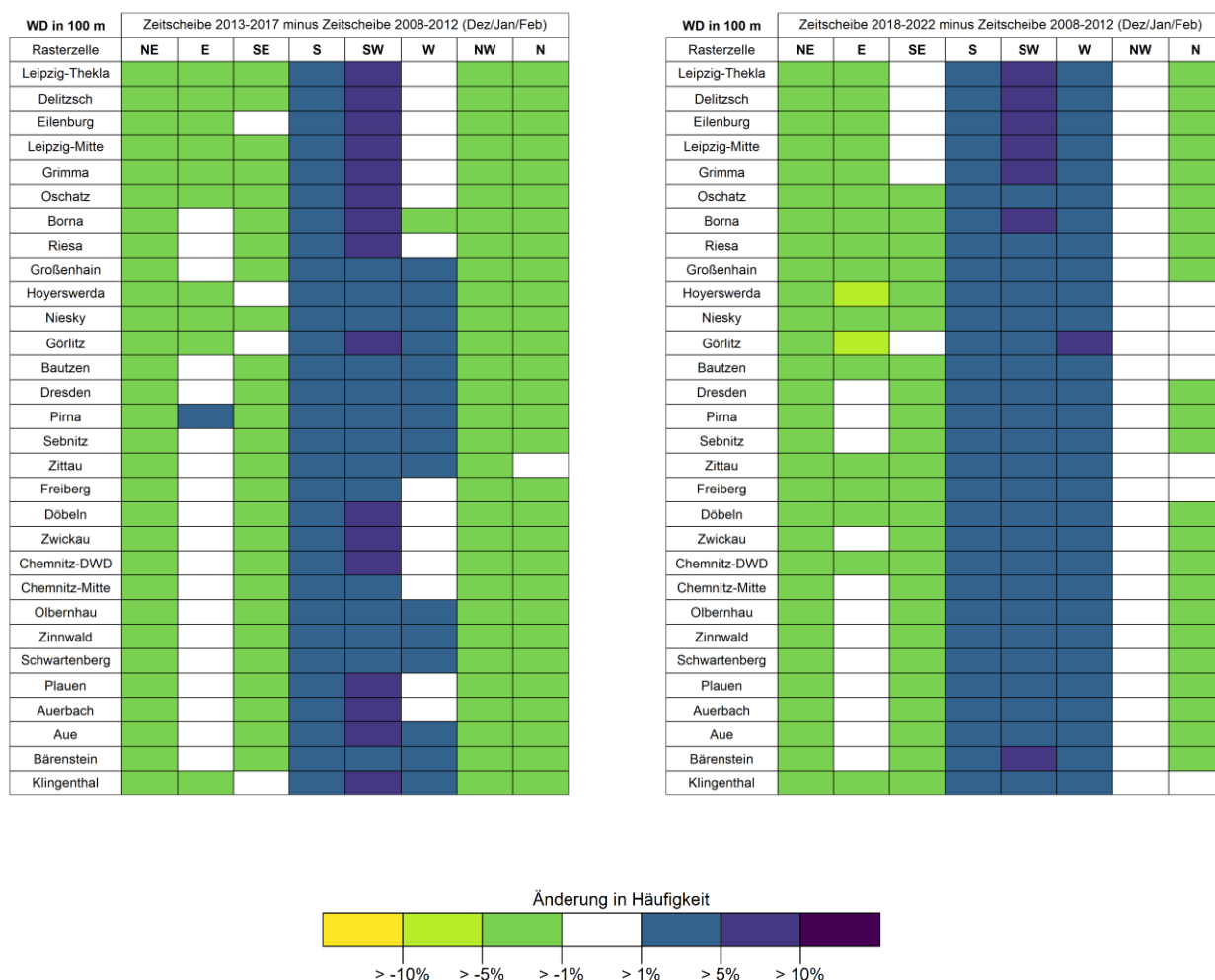
Abbildung 7: Unterschiede in der Windrichtungsverteilung für die Zeitscheibe 2013–2017 (links) sowie 2018-2022 (rechts) in Bezug auf die Zeitscheibe 2008–2012, jeweils für die Monate Dezember, Januar, Februar.
