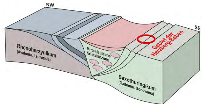
Abb. 5.4-6: Schematische Darstellung der Mitteldeutschen Kristalllinze nach der Kollision der Kontinente Laurussia und Gondwana unter Einbeziehung der Krustensplitter Avalonia (Rhenoharzynikum) und Amorica (Saxothuringikum) im Oberkarbon (nach LINNEMANN et al. 2025).
