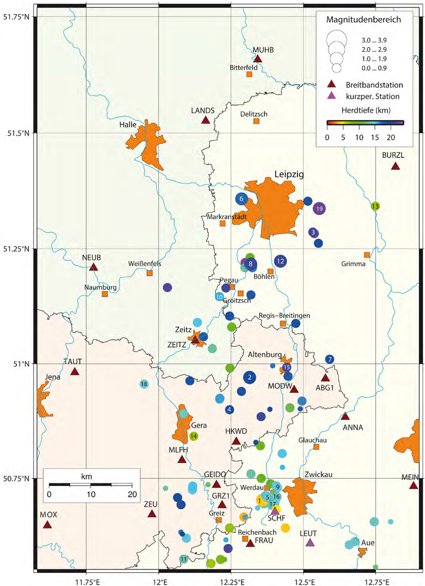
Abb. 2.1-2: Epizentren der Beben im Gebiet nördlich von Plauen bis Leipzig/Halle in den Jahren 2022 bis 2024. Die stärkeren Beben mit M_L \geq 0,7 sind in Tab. 2.1-1 aufgelistet.
