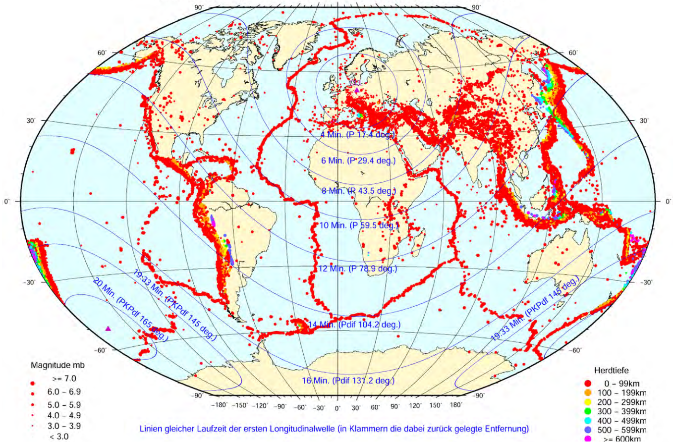
Abb. 5.2-2: Karte der Epizentren der von 2003 bis 2022 in Collm ausgewerteten Erdbeben. Die Herdtiefen sind farblich codiert. Die blauen Linien markieren die Laufzeiten der ersten Welle eines Bebens vom Herd bis nach Collm im 2-Minuten-Abstand.
